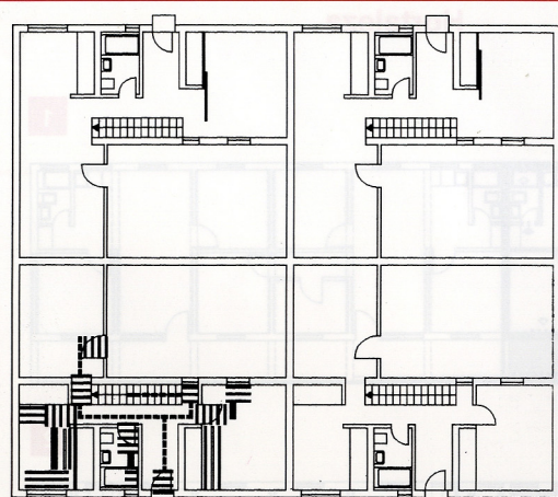
PLANTA BAJA PLANTA ALTA
